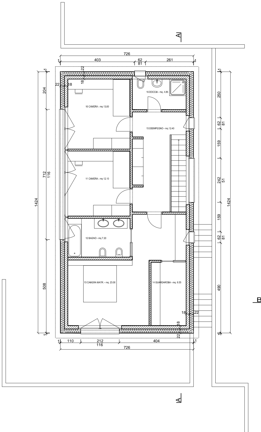
PIANTA PRIMO PIANO 1:100
