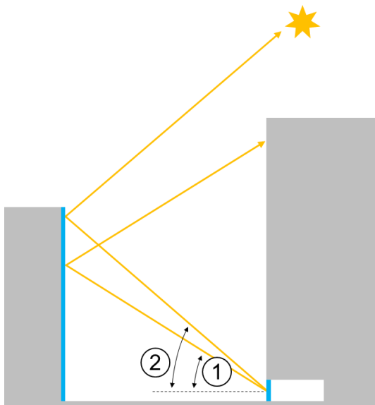
Figura 21: Possibili angoli d'irraggiamento rispettivamente rapporti visivi
