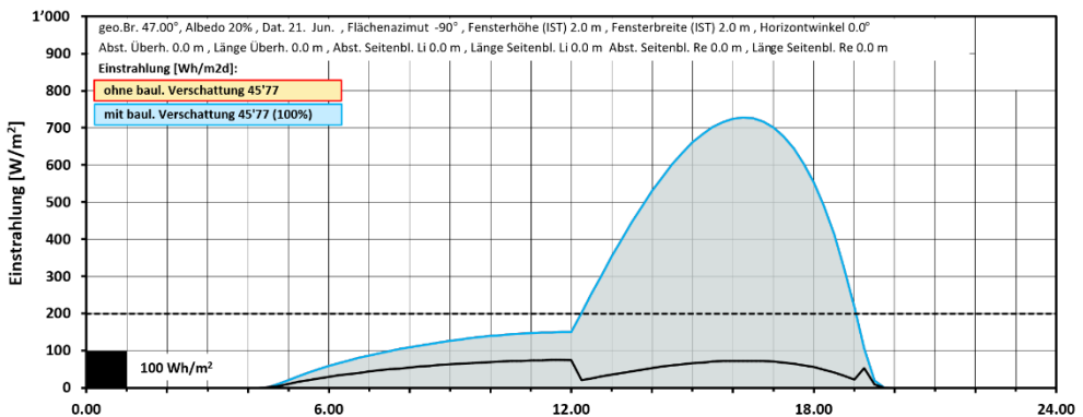
Figure 26 : diagramme d'irradiation ouest le 21 juin
