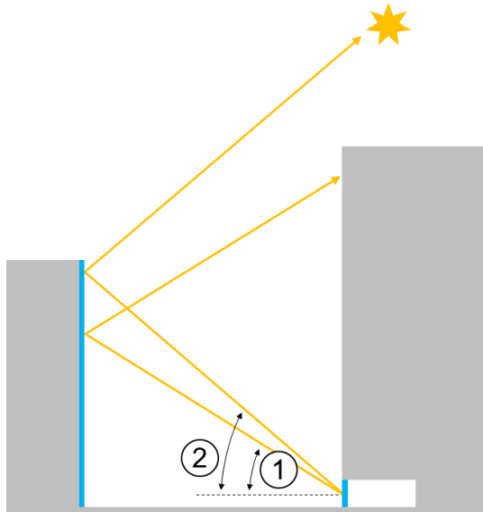
Figure 20: Angles de rayonnement possibles ou éclairage naturel
