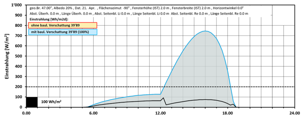
Figure 29 : diagramme d'irradiation ouest le 21 avril
