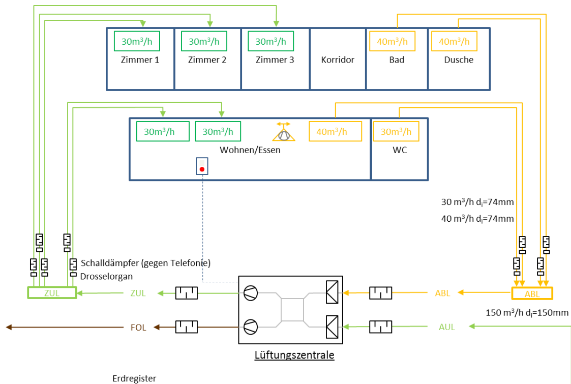
Figure 40: Exemple d'un schéma de ventilation pour les petites installations
