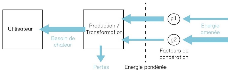
Figure 36 : Schéma de principe du réseau d'énergie
