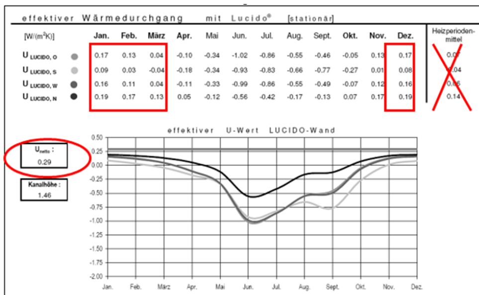
Figure 10 : Spécification de la valeur U pour les façades Lucido
