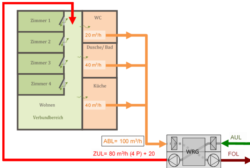
Figure 41 : exemple de ventilation de base pour les rénovations
