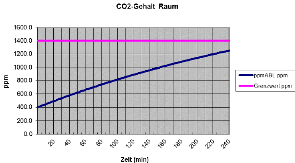
Figure 42 : Teneur en CO 2 pour deux personnes
