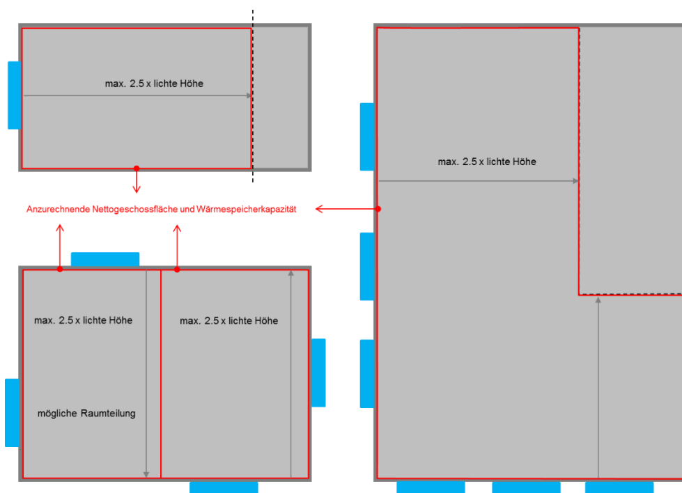
Figure 24: Profondeur maximale imputable et partage des espaces
