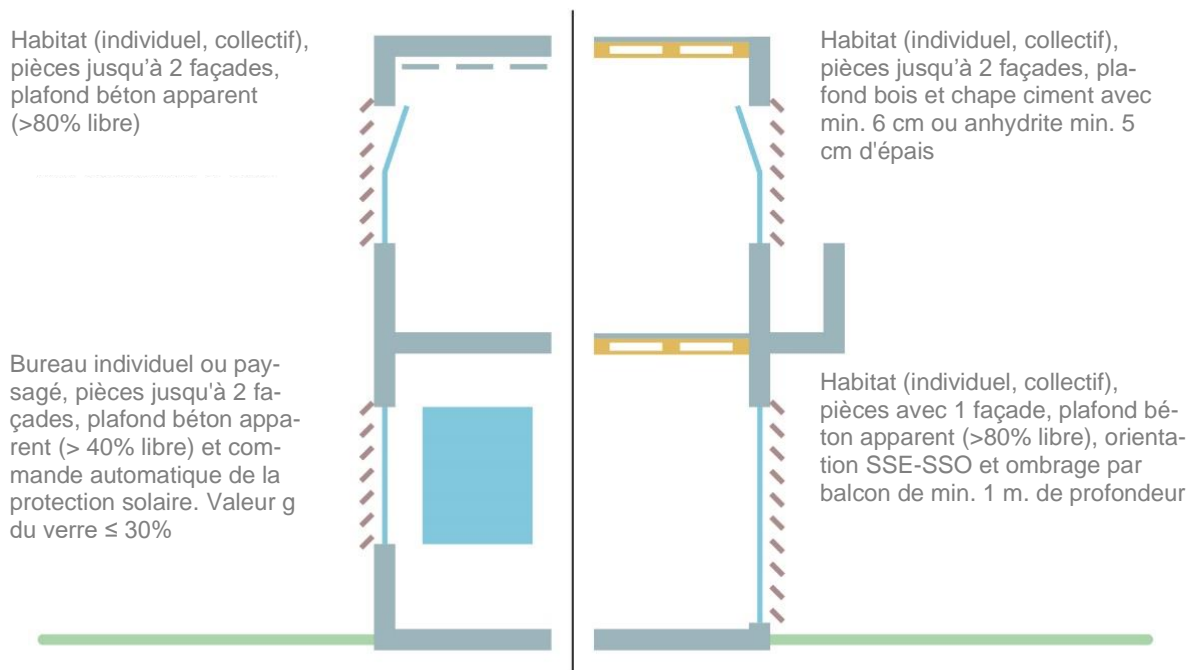
Figure 14: Cas standard pour les bâtiments résidentiels (Variante 1)
