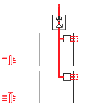
Installation d'extraction d'air avec prises d'air neuf (non autorisé au-delà de 1000 m 3 /h)
