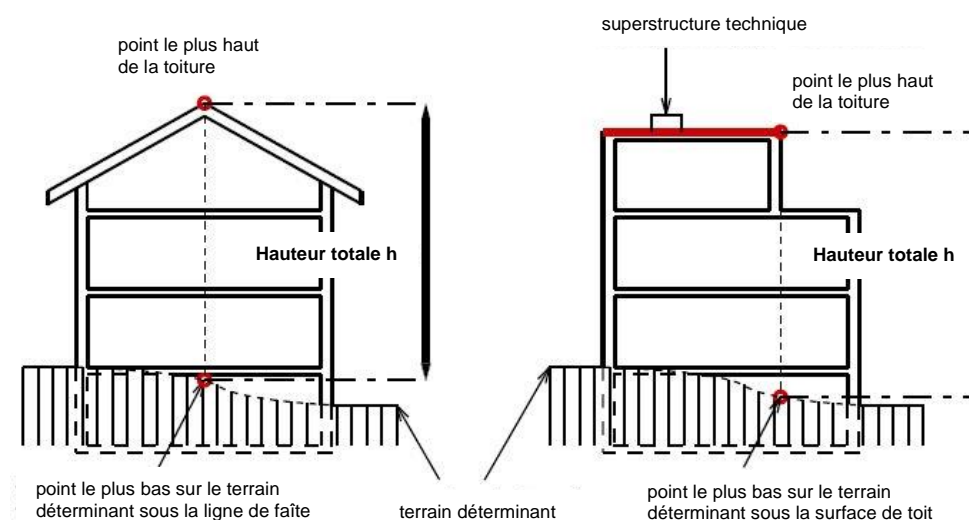
Figure 4 : définition de la hauteur totale du bâtiment
