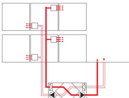
Double flux avec récupération de chaleur (recommandé par Minergie)
