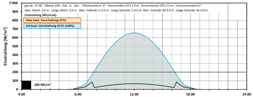
Figure 28 : diagramme d'irradiation sud le 21 avril
