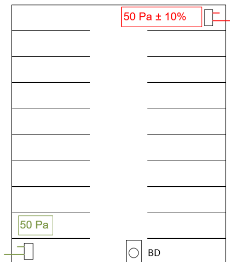
Figura 25 Controllo grafico della differenza di pressione tra interno ed esterno nelle zone critiche
