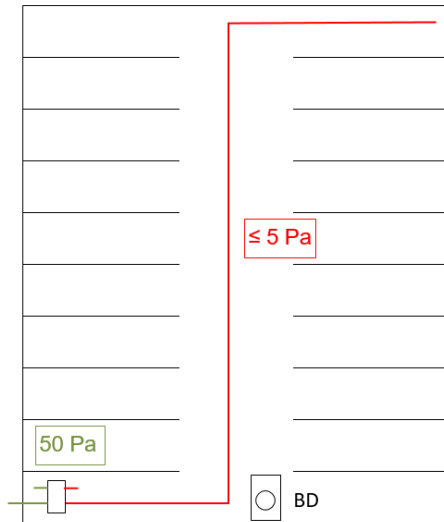
Figura 26 Controllo grafico della differenza di pressione all'interno dell'edificio
