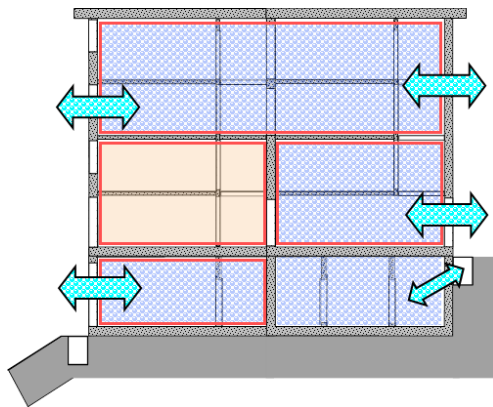
Figura 20 Misurazione di un'unità d'uso (appartamento) in un edificio (abitazione PF). Le finestre degli appartamenti confinanti, della scala e dei locali adiacenti non riscaldati vanno aperte
