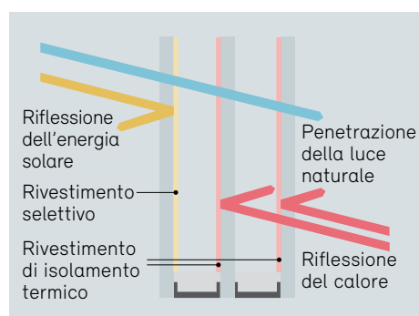
Struttura di un vetro con protezione solare.
