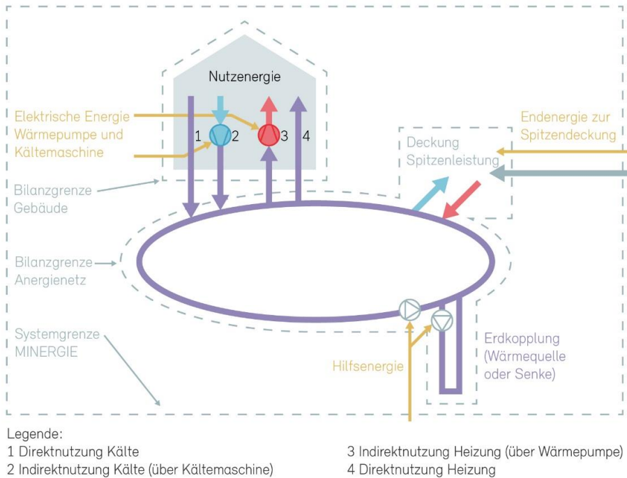
Abbildung 36: Prinzipskizze Anergienetz
