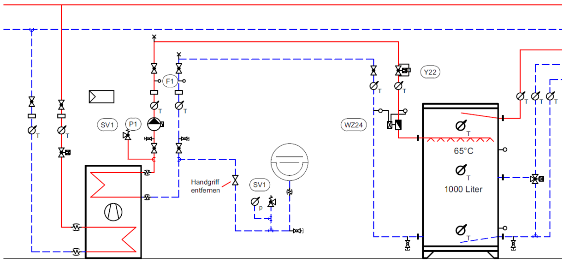
Abbildung 38: Schema Warmwasser-Booster
